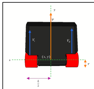
Figura 1. Cinemática de un robot mini sumo.
