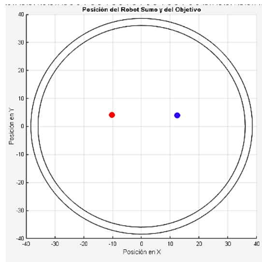
Figura 6. Simulación del mini sumo 2.
