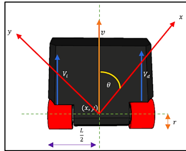
Figura 3. Movimientos del robot mini sumo.
