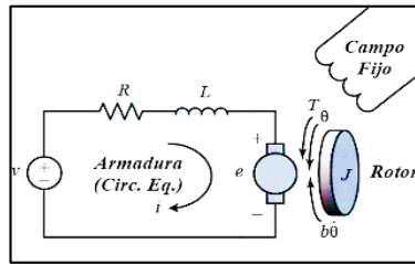
Figura 2. Representación eléctrica del motor.
