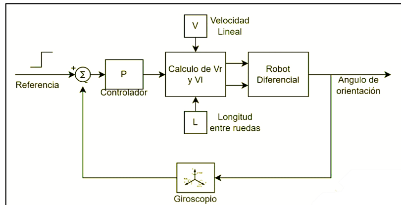
Figura 4. Diagrama de bloque del mini sumo.
