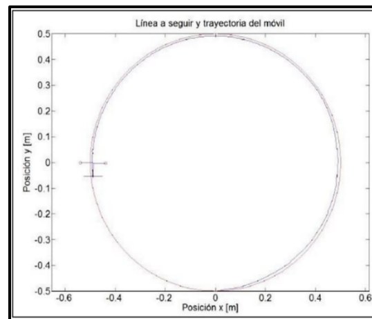
Figura 9. Grafica del recorrido del robot
