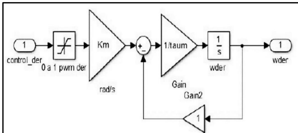
Figura 7. Control de motor derecho
