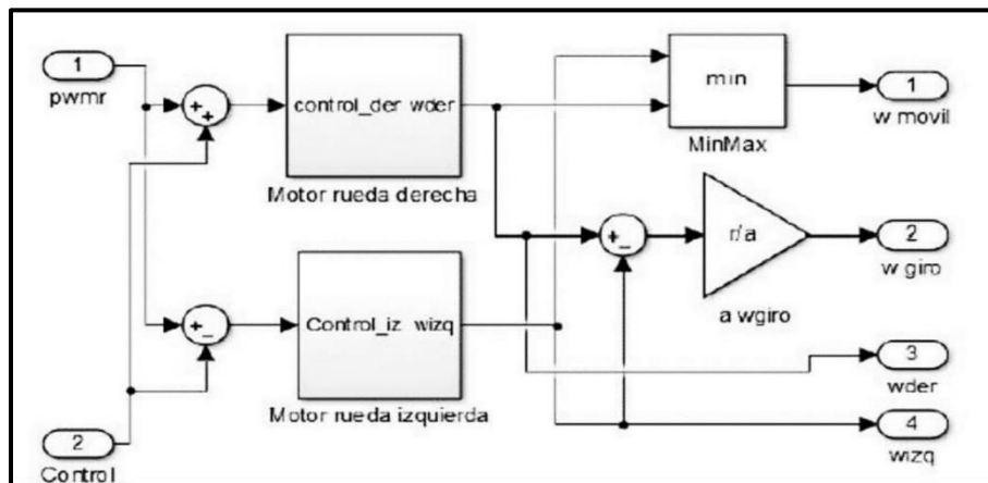
Figura 5. Control de los motores
