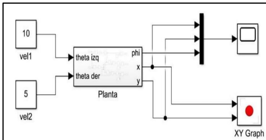
Figura 3. Diagrama del robot en Simulink
