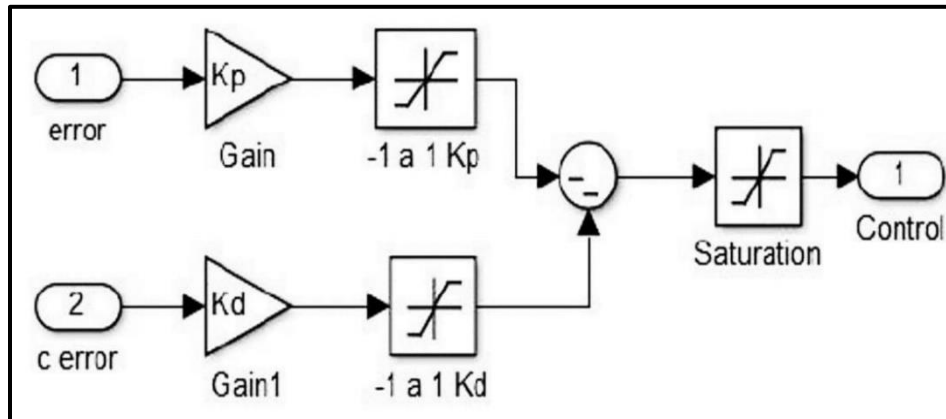
Figura 6. Valores de KP Y KD
