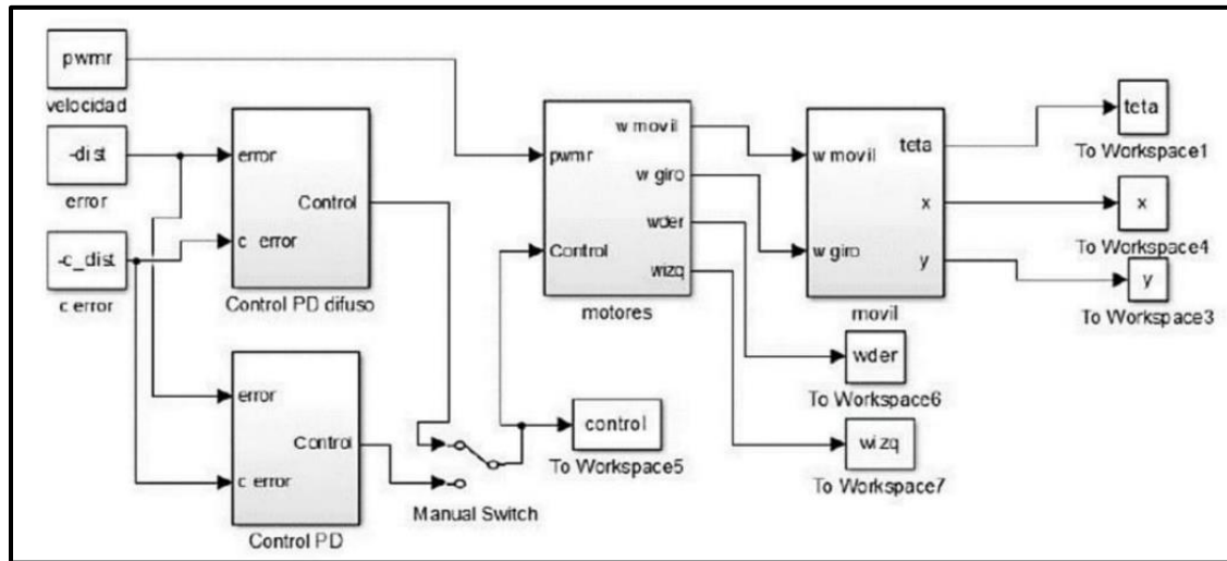
Figura 4. Error y PD
