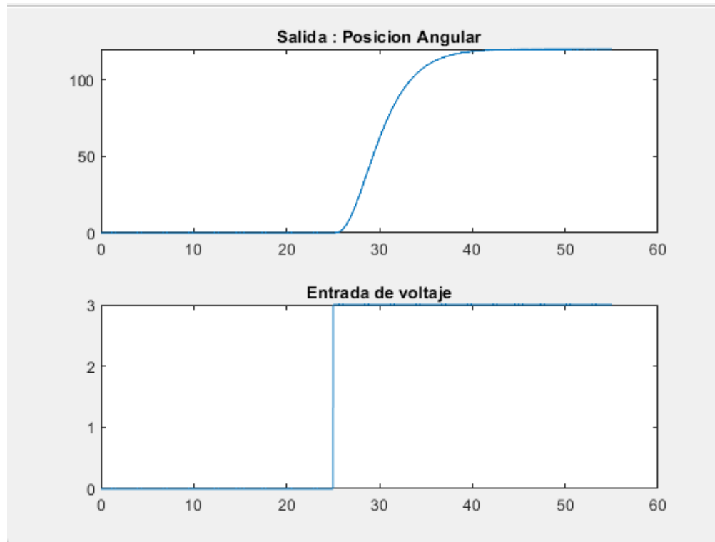
Figura 1: Entrada y Salida de mi sistema lineal.
