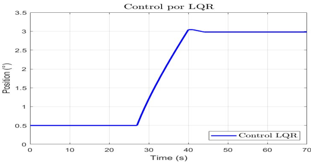
Figure 11: Control por regulador cuadrático lineal (LQR)
