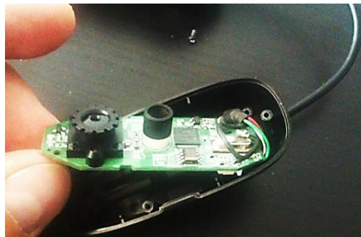
Figura 2. Circuito físico de la cámara Logitech C270
