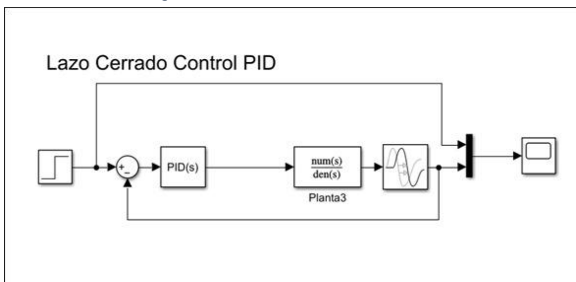
Figura 1. Control en lazo cerrado utilizado para auto sintonización
